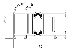
Profil ościeżnicy ALU/75
