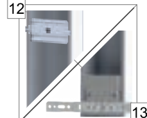
12 Elementy wzmacniające konstrukcję ościeznicy z kotwami montażowymi lub bez 12. Ościeznica 10/54,11/54 13. Ościeznica 15/54
