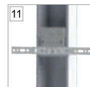
11 Elementy wzmocniające konstrukcję ościeżnicy z kotwami montażowymi
