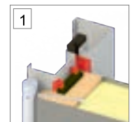
Wypełnienie skrzydła PIANA POLIURETANOWA
