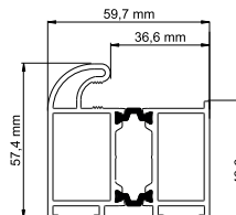
Profil ościeżnicy ALU/54
