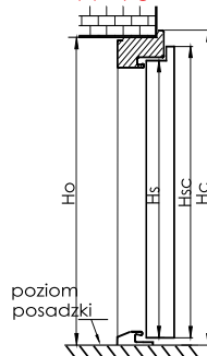
Drzwi trzy przylgowe 3P
