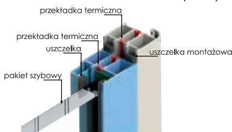
PROFIL NAŚWIETLA PROFIL OŚCIEŻNICY ALU/54
