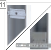
11 Elementy wzmacniające konstrukcję ościeżnicy z kotwami montażowymi lub bez 12. Ościeżnica 10/54, 11/54 12. Ościeżnica 15/54
