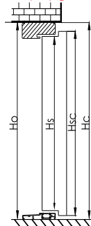
Drzwi cztero przylgowe 4P
