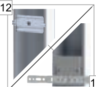
12, 13 Elementy wzmacniające konstrukcję ościeżnicy z kotwami montażowymi lub bez 12. Ościeżnica 10/54,11/54 13. Ościeżnica 15/54
